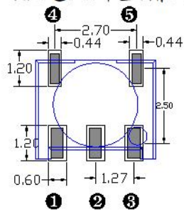
正贴建议焊盘排列一
