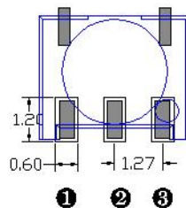
正贴建议焊盘排列二
