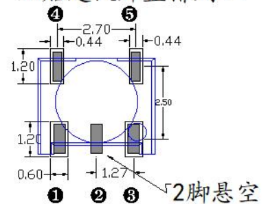
正贴建议焊盘排列三
