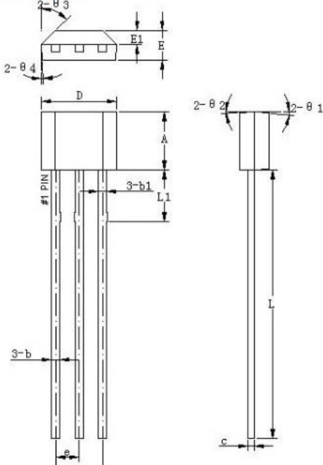
TO-92S-A1/A2 TO-92S-A1
