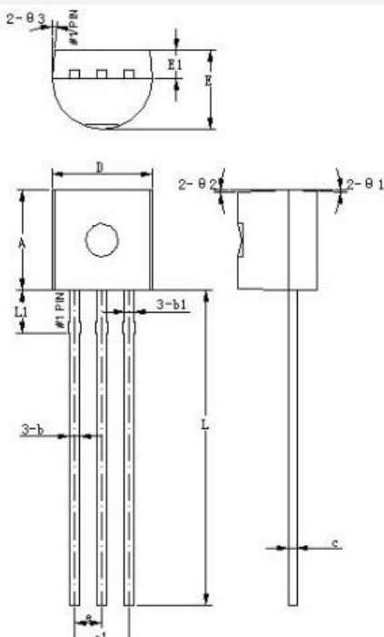
TO-92-A1
