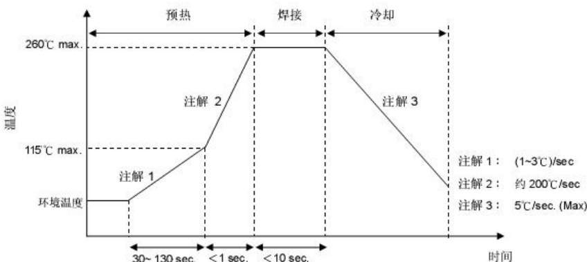
波峰焊接曲线
