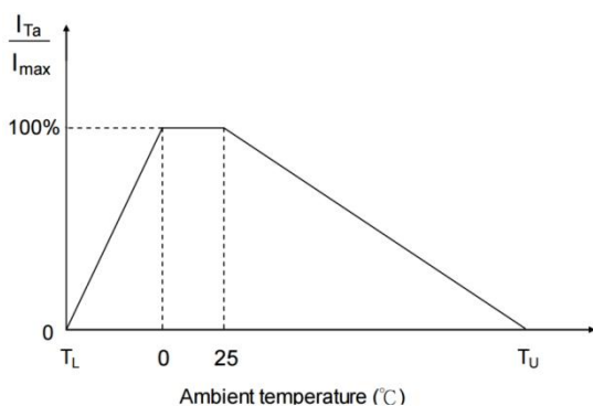
■ 最大电流降额曲线图
