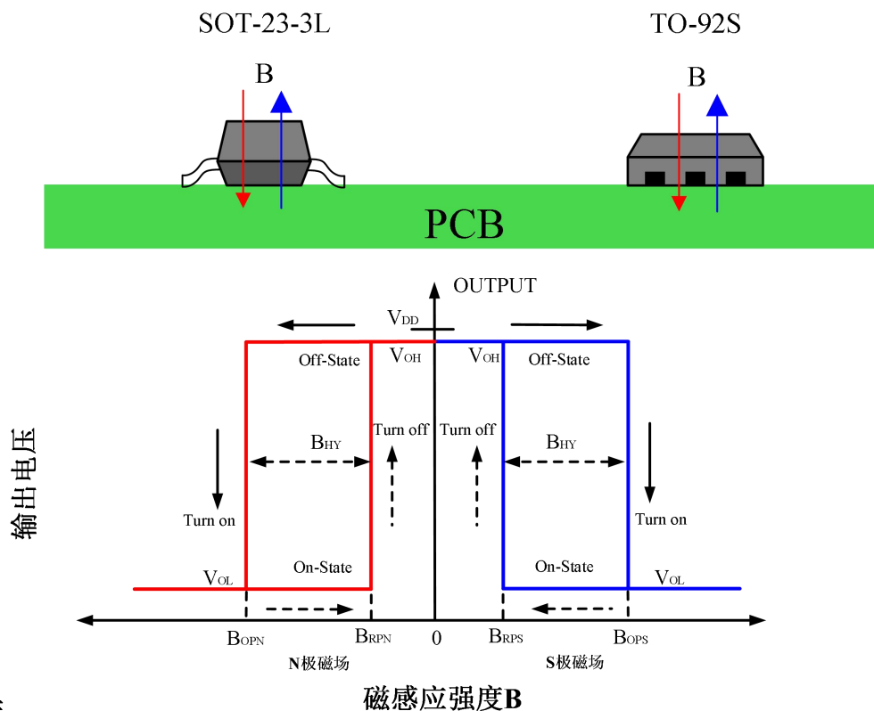
输出特性
