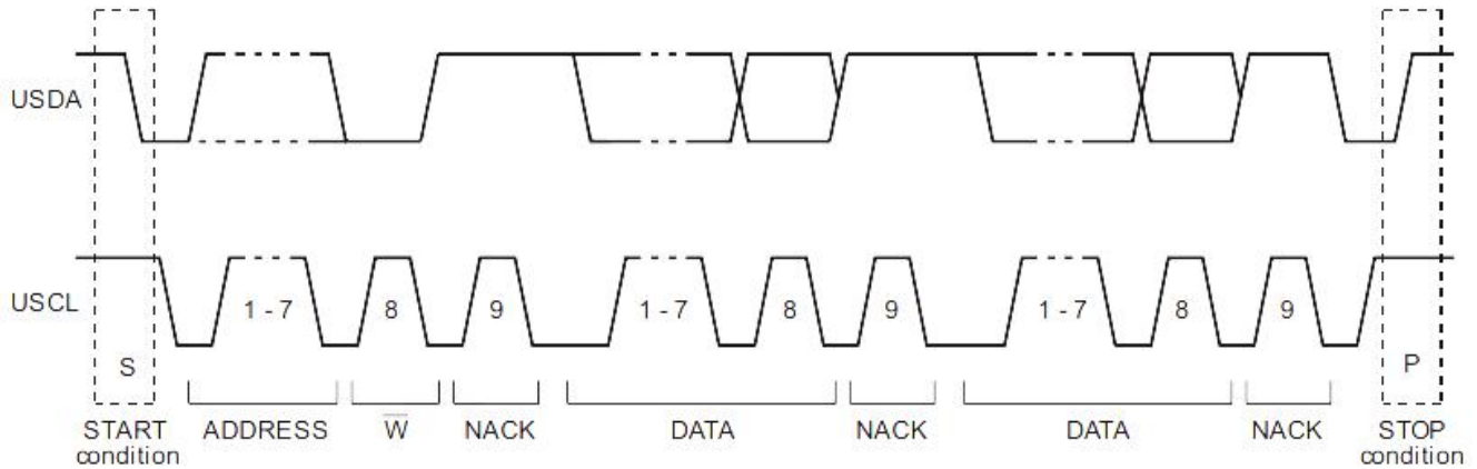
图 4. I2C 通讯协议
