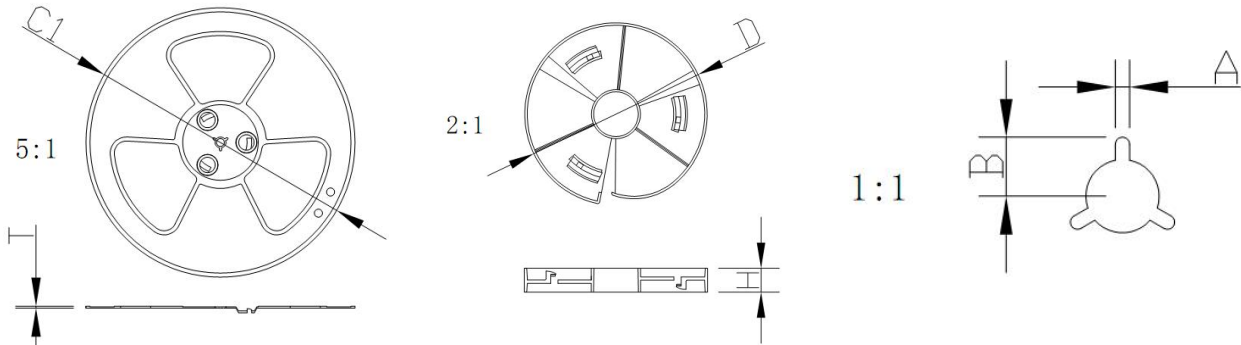
图 10. 卷盘规格
