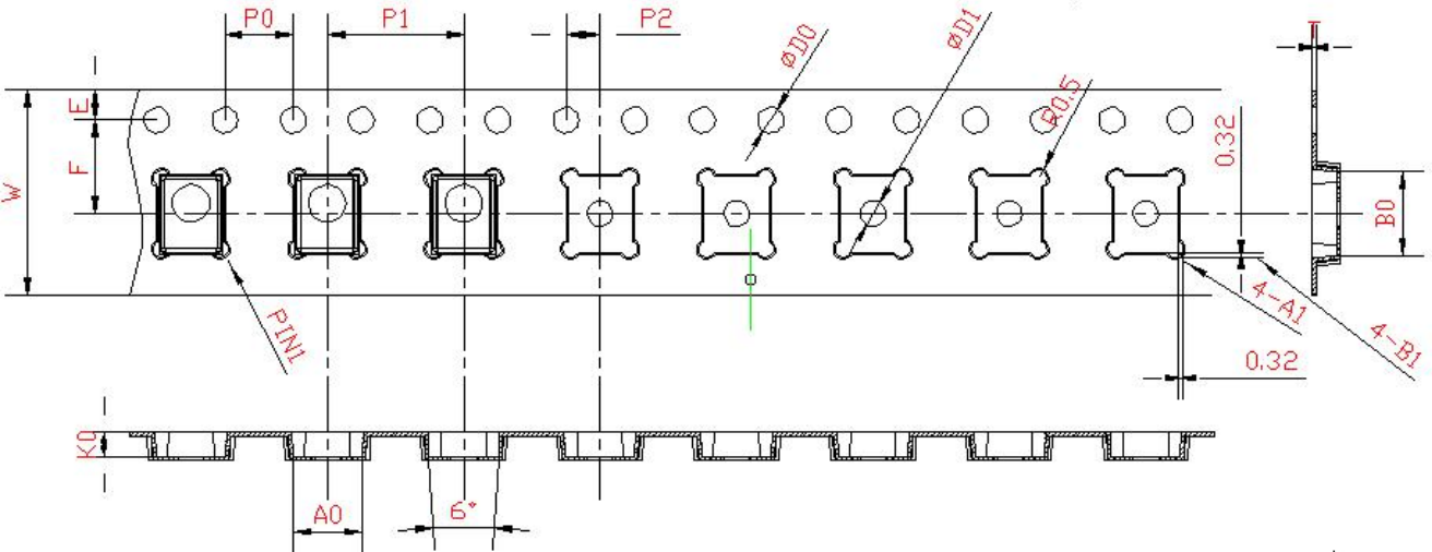
图 9. 载带规格
