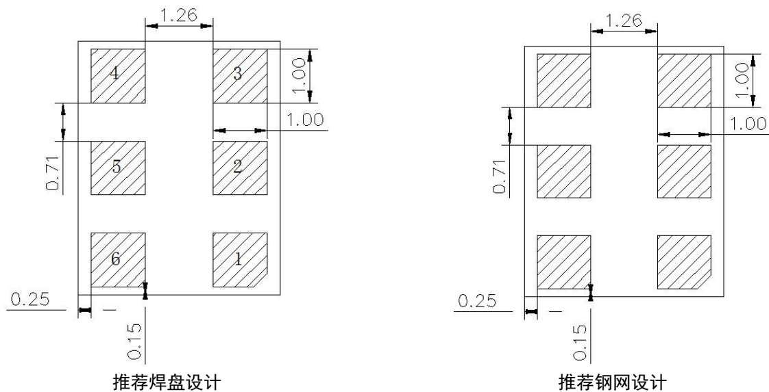
图 7. 推荐焊盘与钢网设计 (单位: mm)
