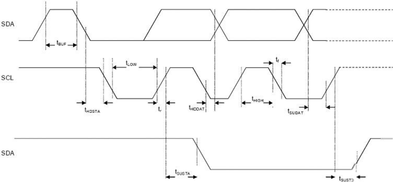
图 3. I2C 时序图
