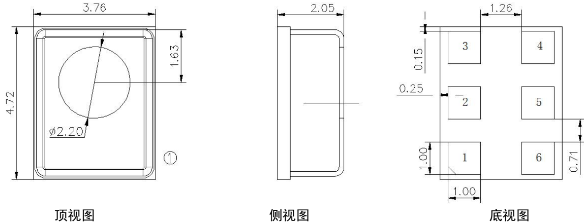
图 6. 轮廓尺寸
